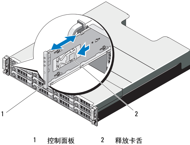
图 16-13. 卸下和安装控制面板 -PowerVault MD3600f
